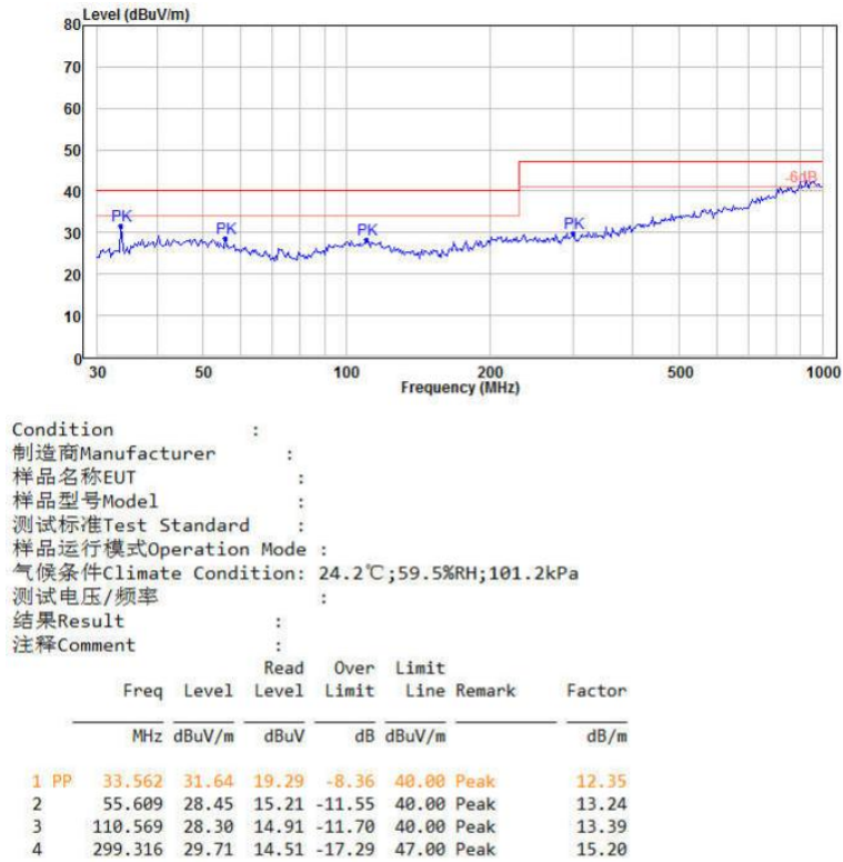
图 6-6 RE 测试垂直方向
