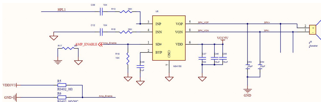
图 3-3 音频参考电路
