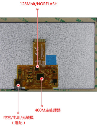
图 1-4 硬件配置图
